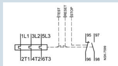
Relé de sobrecarga 3RU11 2 hasta 3RU11 4
