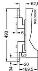
Conexión vertical, hasta 6300 A
