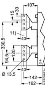
Conexión vertical
