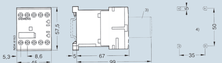
Contactores 3RT10 y 3RH11 Tamaño S00
