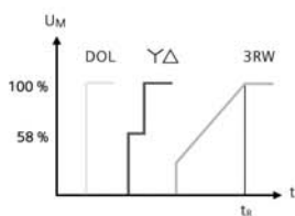
Comparación de diferentes tipos de arrancadores: arranque directo, Y-triángulo* y arranque suave
