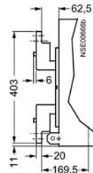
Conexión frontal (doble hilera de perforaciones) según DIN 43 673, hasta 4000 A
