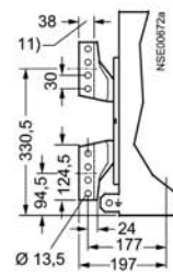
Conexión plana, hasta 4000 A
