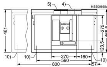
Ejecución estándar Conexión horizontal, hasta 5000 A
