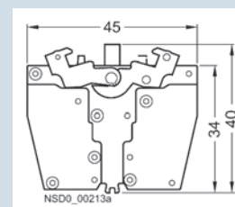
Bloque de contacto 2 elementos
