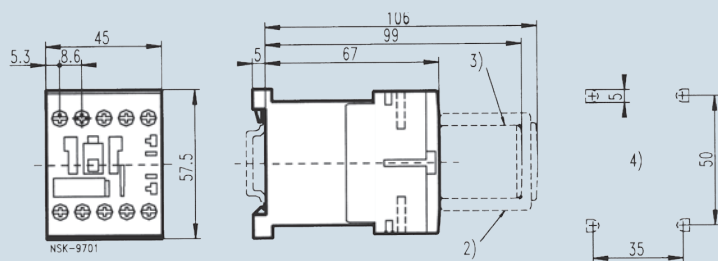
Contactores auxiliares 3RH Tamaño S00, conexión por tornillo con limitador de sobretensión bloque de contactos auxiliares
