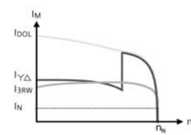
Comparación de diferentes tipos de arrancadores: arranque directo, Y-triángulo* y arranque suave
